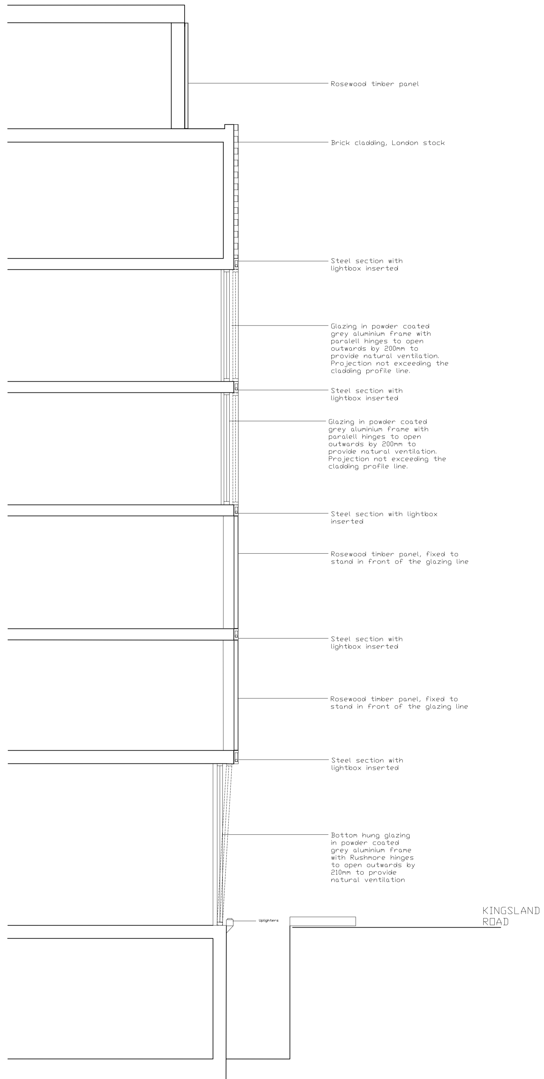
Section A1- A1
